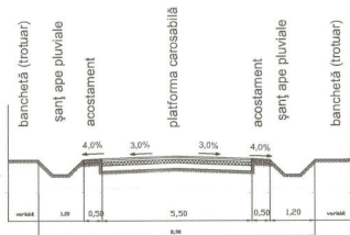
Secțiune caracteristică străzi reabilitate, 4,00 m
